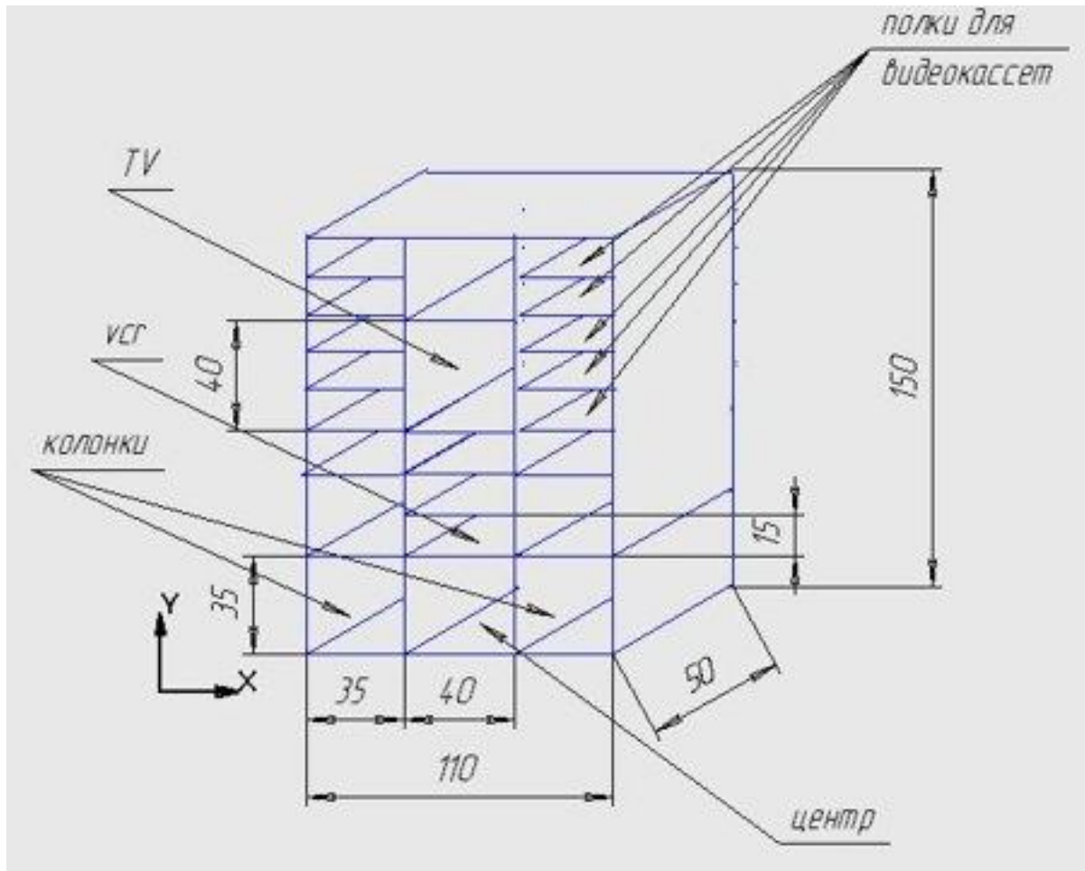
Рис. 1. Эскиз заказчика.
